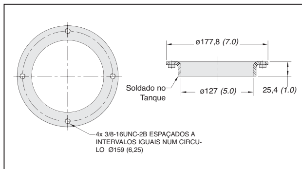
Dimensões em mm (polegada)
